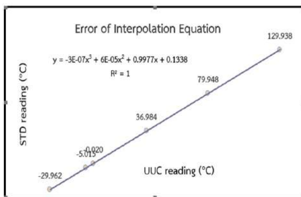
ภาพ 12 กราฟแสดงค่าสมการ polynomial (y) จากผลการสอบเทียบ data logger with PRT ID No.CALT_T01(109)
