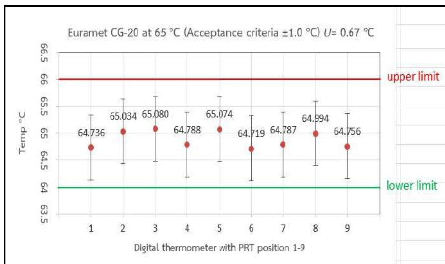
ภาพ 25 ผลการทวนสอบ 9 ตำแหน่งจากผลการสอบเทียบตู้บ่มเพาะเชื้อ S/N: 20230000001553 ตามวิธี EURAMET CG-20 จุดสอบเทียบ 65 °C ที่ acceptance criteria เท่ากับ \pm 1.0 °C
