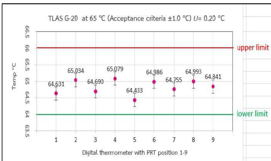
ภาพ 19 ผลการทวนสอบ 9 ตำแหน่งจากผลการสอบเทียบตู้บ่มเพาะเชื้อ S/N: 20230000001553 ตามวิธี TLAS G-20 จุดสอบเทียบ 65 °C ที่ acceptance criteria เท่ากับ \pm 1.0 °C
