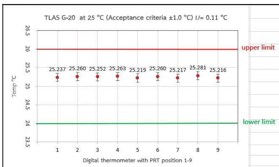
ภาพ 14 ผลการทวนสอบ 9 ตำแหน่งจากผลการสอบเทียบตู้บ่มเพาะเชื้อ S/N: 20190000013001 ตามวิธี TLAS G-20 ที่จุดสอบเทียบ 25 °C acceptance criteria เท่ากับ \pm 1.0 °C
