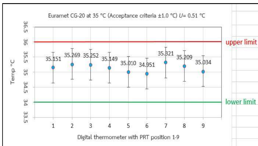
ภาพ 22 ผลการทวนสอบ 9 ตำแหน่งจากผลการสอบเทียบตู้บ่มเพาะเชื้อ S/N: 12-18771 ตามวิธี EURAMET CG-20 จุดสอบเทียบ 35 °C ที่ acceptance criteria เท่ากับ \pm 1.0 °C
