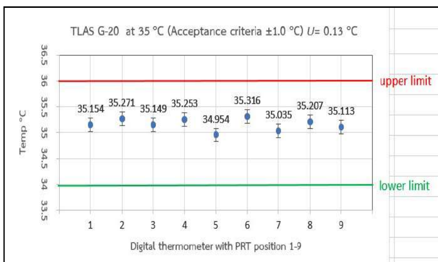
ภาพ 16 ผลการทวนสอบ 9 ตำแหน่งจากผลการสอบเทียบตู้บ่มเพาะเชื้อ S/N: 12-18771 ตามวิธี TLAS G-20 จุดสอบเทียบ 35 °C ที่ acceptance criteria เท่ากับ \pm 1.0 °C
