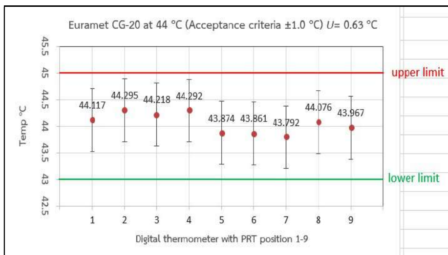
ภาพ 24 ผลการทวนสอบ 9 ตำแหน่งจากผลการสอบเทียบตู้บ่มเพาะเชื้อ S/N: 04-92541 ตามวิธี EURAMET CG-20 จุดสอบเทียบ 44 °C ที่ acceptance criteria เท่ากับ \pm 1.0 °C
