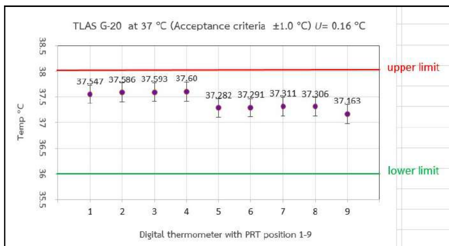
ภาพ 17 ผลการทวนสอบ 9 ตำแหน่งจากผลการสอบเทียบตู้บ่มเพาะเชื้อ S/N: 04-66267 ตามวิธี TLAS G-20 จุดสอบเทียบ 37 °C ที่ acceptance criteria เท่ากับ \pm 1.0 °C
