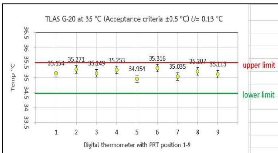
ภาพ 15 ผลการทวนสอบ 9 ตำแหน่งจากผลการสอบเทียบตู้บ่มเพาะเชื้อ S/N: 12-18771 ตามวิธี TLAS G-20 ที่จุดสอบเทียบ 35 °C acceptance criteria เท่ากับ \pm 0.5 °C
